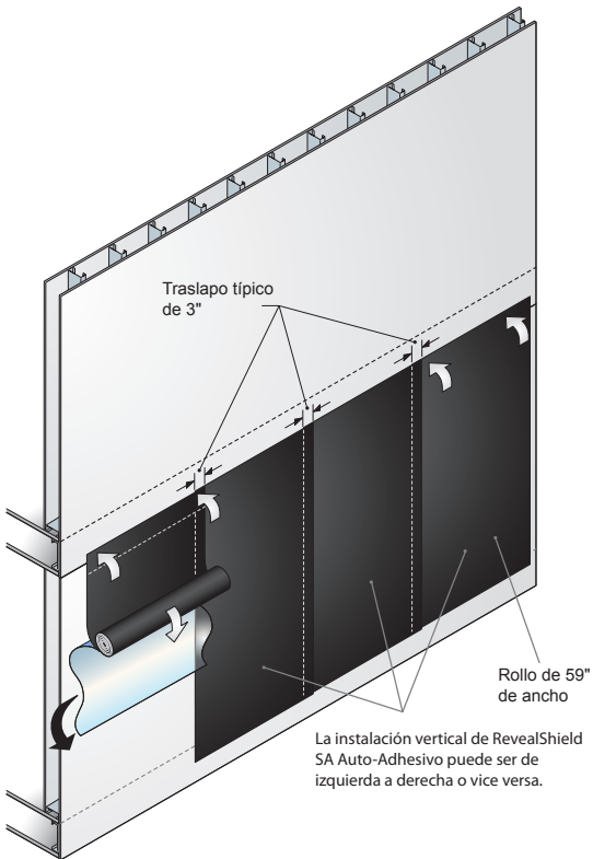
INSTALACIÓN VERTICAL
