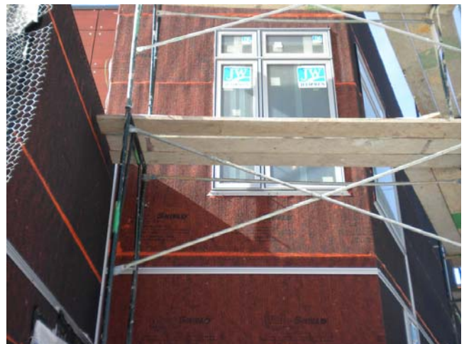
WrapShield HS under stucco.
